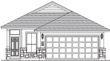
ELEVATION A
